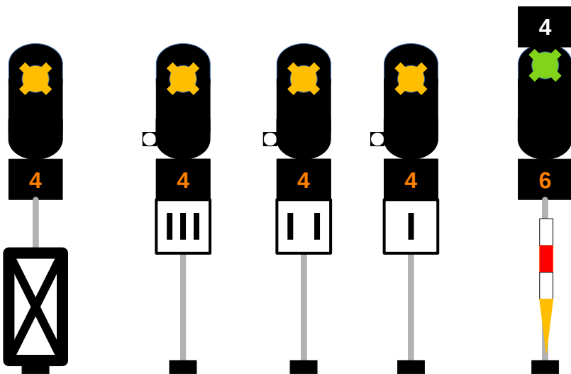
d) Semafor wjazdowy wyświetla sygnał S3 „jazda z W21b”, dodatkowo świeci się wskaźnik W21a.
